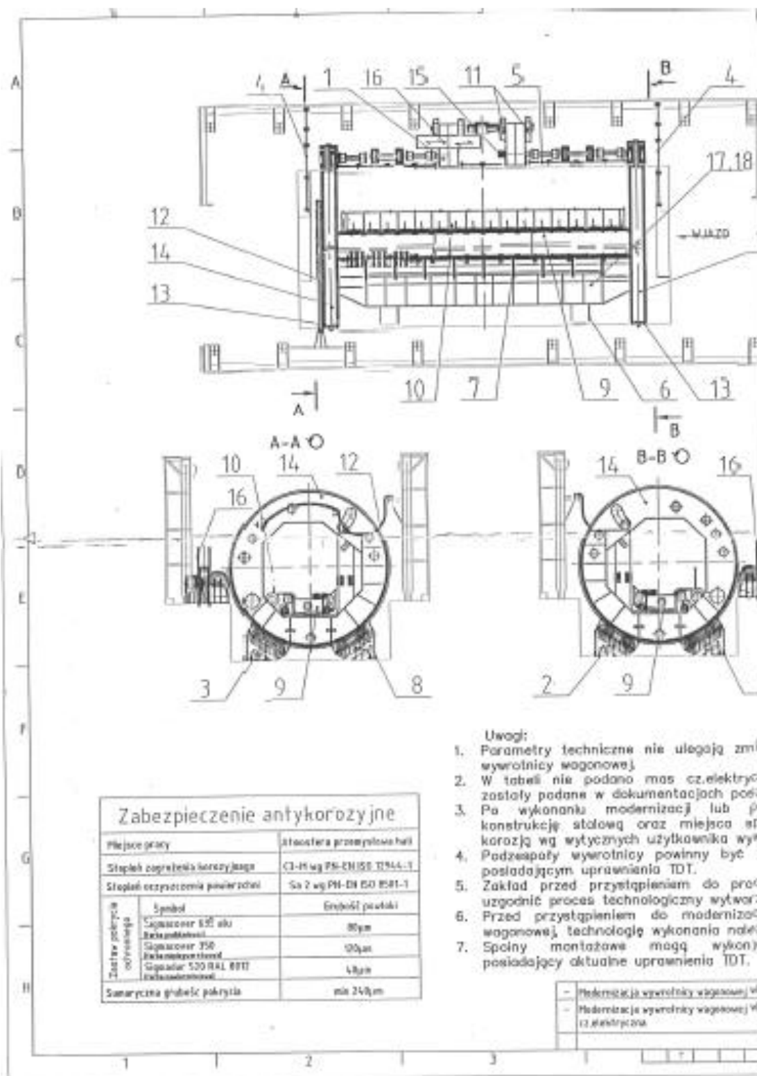
Załącznik nr 3 do SIWZ – WW1 – Widok ogólny wywrotnicy wagonowej
